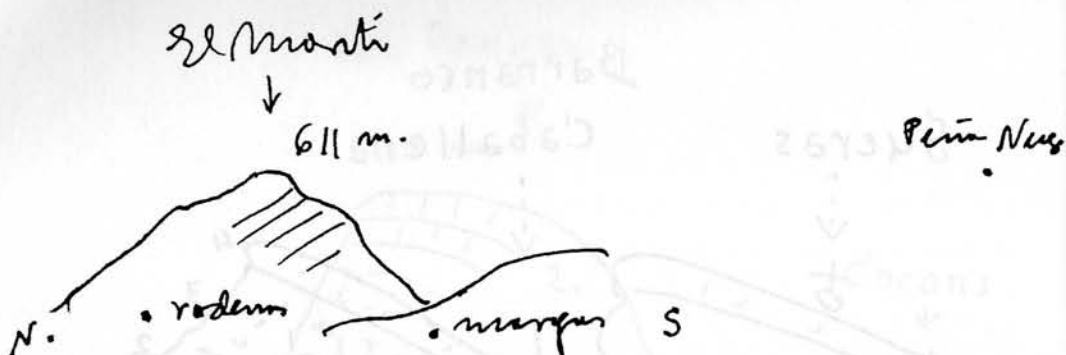
Figura 25. Antes de llegar a Tales desde Eslida. Sin escala.
