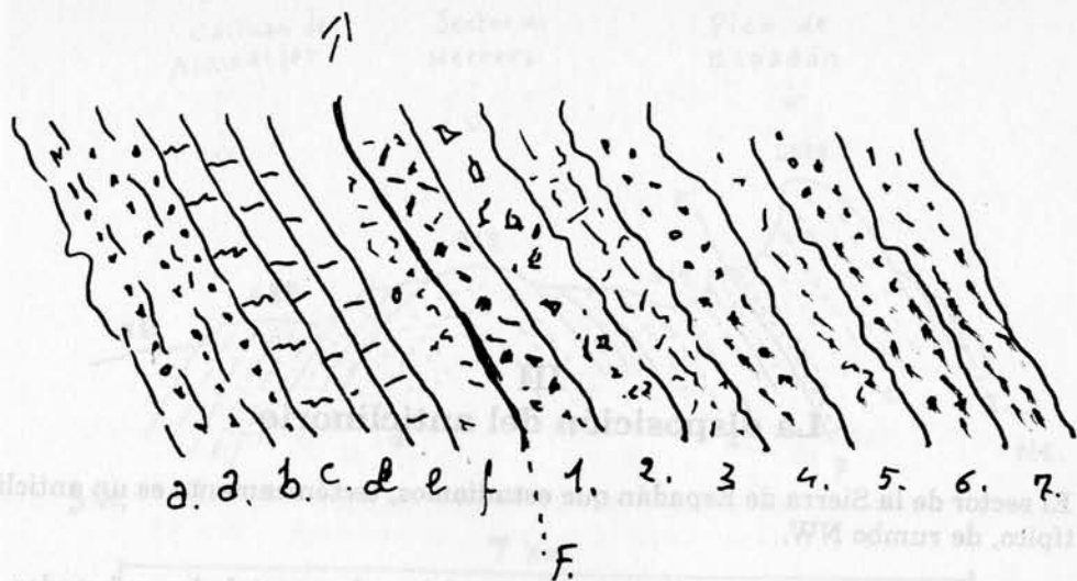
Figura 6. Contacto anormal y milonito comprobable en el trayecto de Almedijar a Ahín. F. Zona de contacto anormal, superficie de cabalgamiento. — 1. Calizas munchselkalk, brechoides, milonitizadas, grises y zona de fricción. — 2. Brecha con cemento amarillo, fragmentos de areniscas arcillosas, rojas, verdes, fragmentos de calizas. — 3. Zona de areniscas margosas rojo-oscuras, muy milonitizadas, con intercalaciones de cuarzo en vetas lechosas. — 4. Capa de rodenos rojos, areniscas típicas, resquebrajados. — 5. Rodenos como los anteriores más difusos. — 6. Areniscas típicas, amarillentas, fracturadas. — 7. Rodenos típicos. — a. Areniscas, rodenos típicos de transición al Muschelkalk. — b. Areniscas, rodenos de transición. — c. Calizas del Muschelkalk. — d. Calizas del Muschelkalk afectadas por presiones. — e, f. Capas de calizas afectadas por el resbalamiento.
