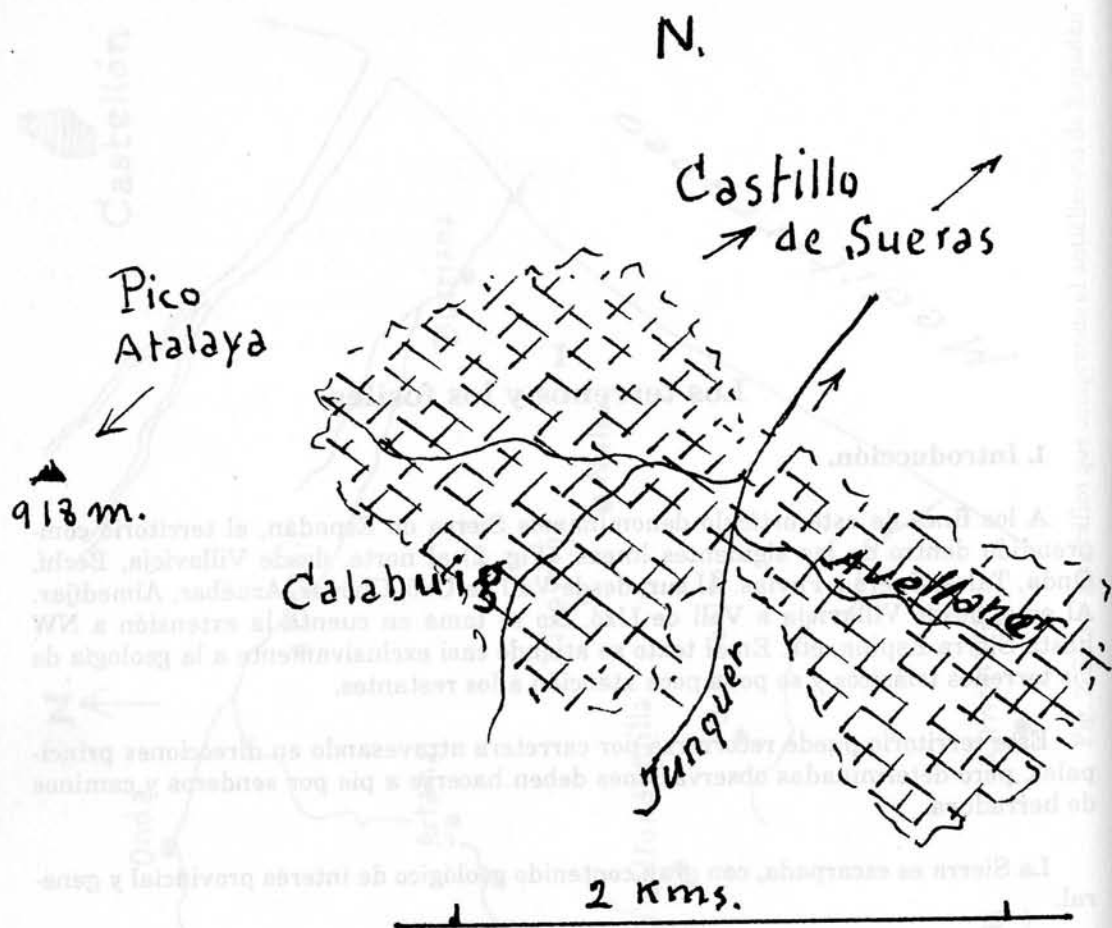
Fig. 3. Paleozoico del paraje llamado Pedralba al W de Sueras
