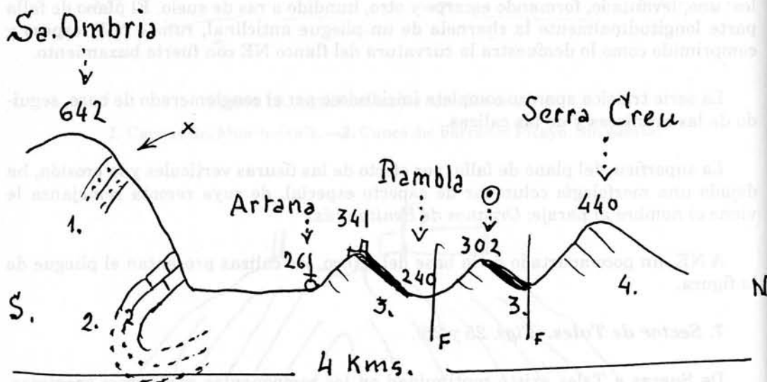
Figura 22. Perfil geológico de Artana. Sin escala.
