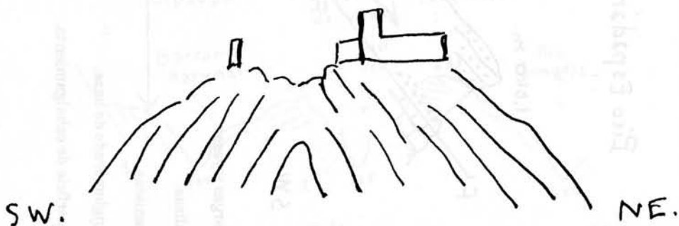
Figura 20. Pliegue anticlinal en el castillo de Ahín. Charnela en calizas del Muschelkalk, con eje de rumbo NNW a SE, se continua con la charnela de la Font de Caritat y a NW se prolonga hacia la base del Pico de Espadán. Sin escala.
