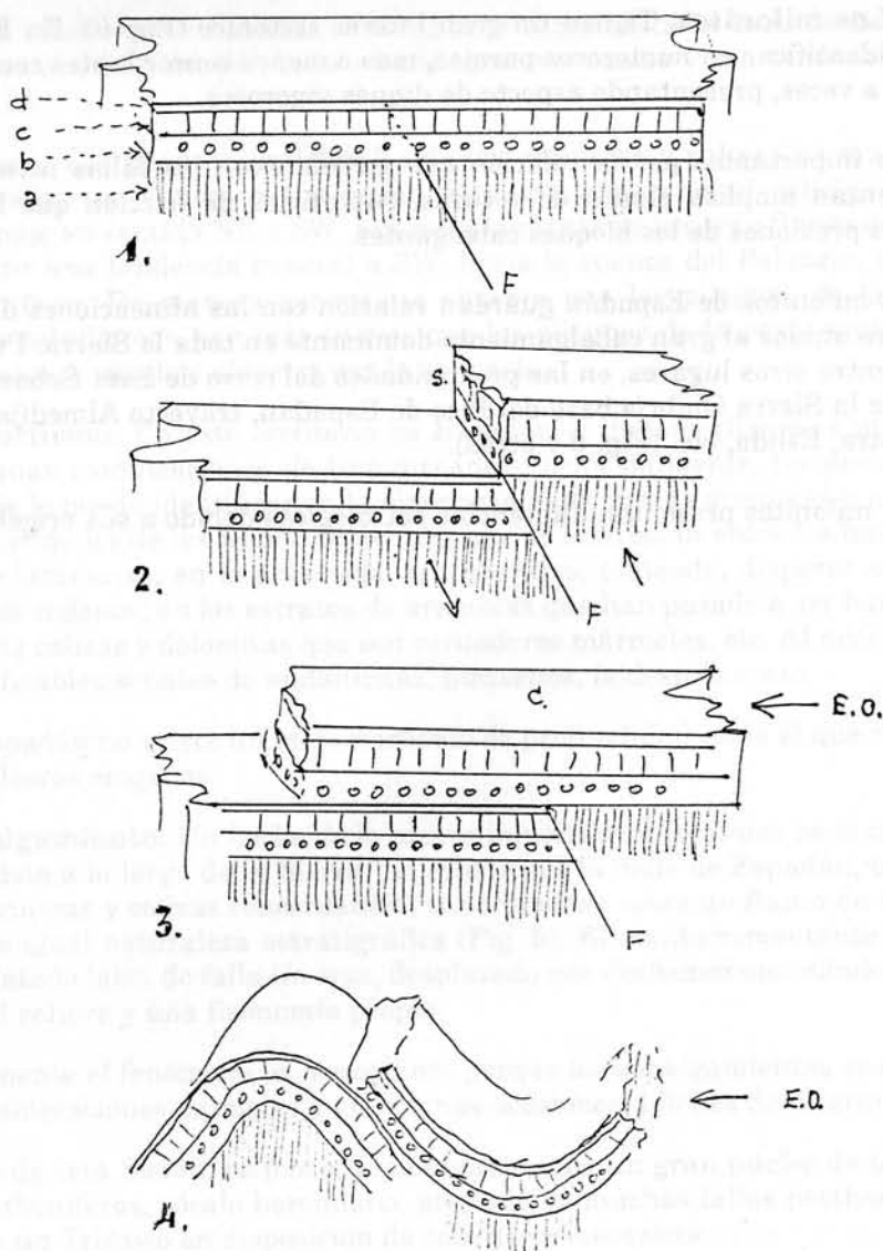
Figura 5. Interpretación del cabalgamiento.
