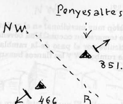
Figura 28. Anticlinal Penyes Altes de rumbo NW, partido por la charnela R , rambla de Artana.
