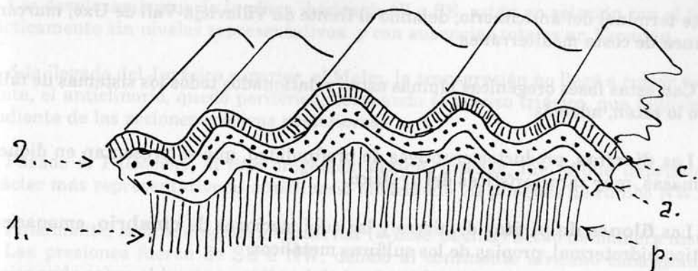
Figura 35. Corte teórico en anticlinorio de la orogenia alpina.
