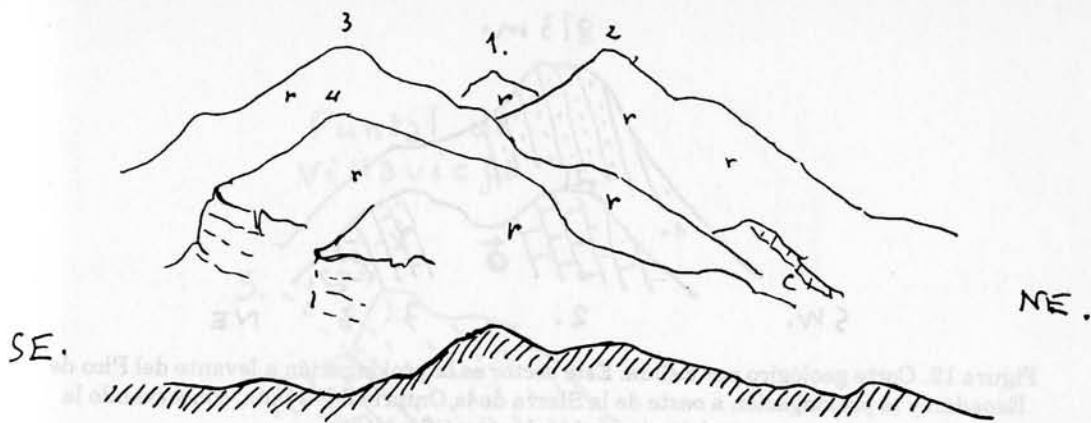
Figura 10. Panorámica del relieve central del anticlinorio de Espadán, de cumbres alineadas de SE a NW. Morfología del relieve en la línea central de la Sierra.
