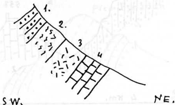
Figura 14. Contacto de la estratificación invertida en Jorva.
