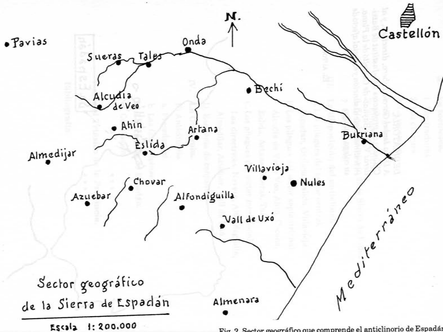
Fig. 2. Sector geográfico que comprende el anticlinorio de Espadán
