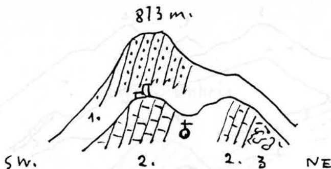
Figura 12. Corte geológico por Eslida. Este sector es la prolongación a levante del Pico de Espadán y la prolongación a oeste de la Sierra de la Ombría de Artana, conservando la posición invertida de estratificación.
