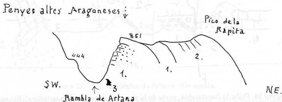
Figura 27. Flanco de anticlinal partido. Sin escala.
