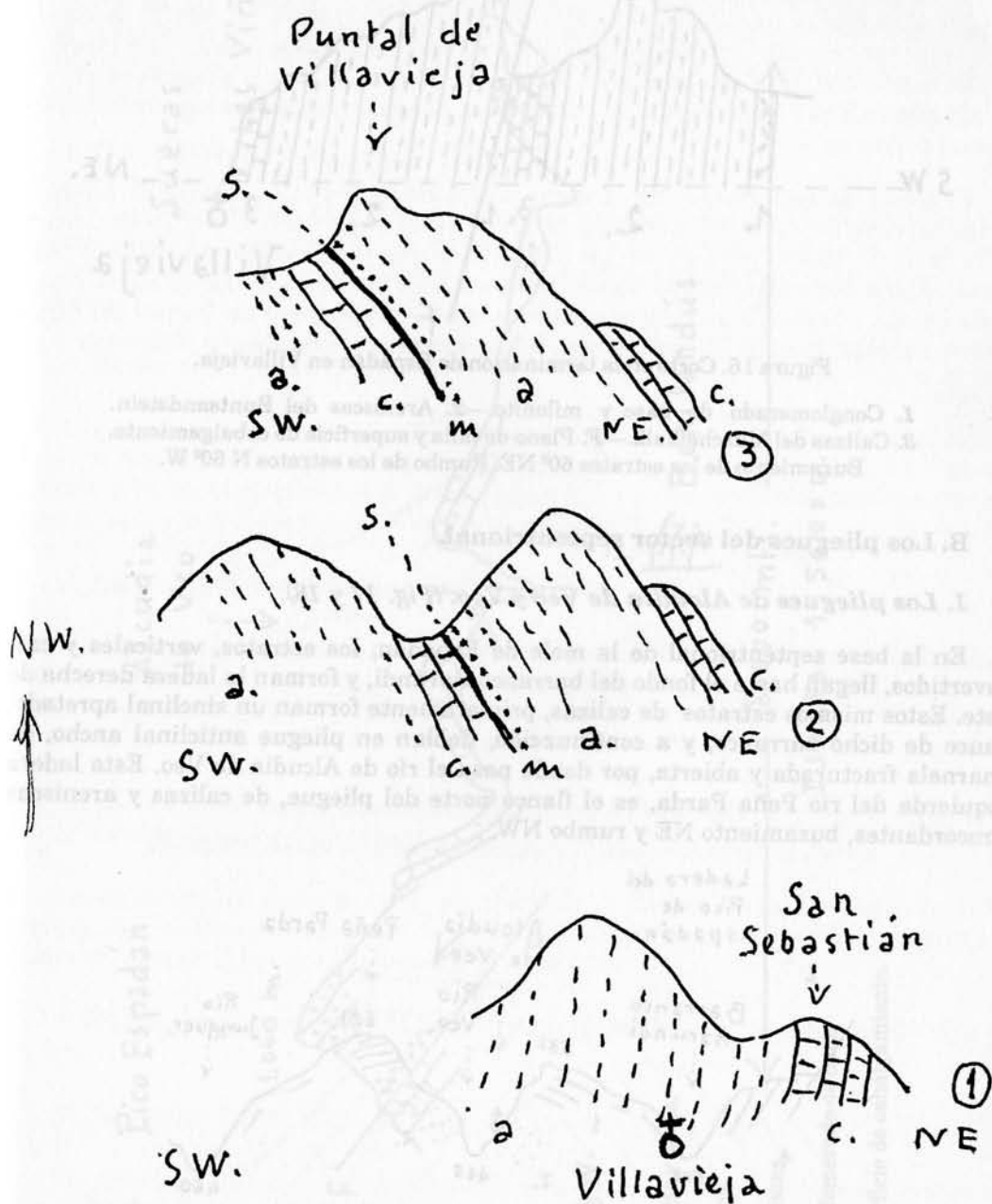
Figura 15. Cabalgamiento en el Puntal de Villavieja. En Villavieja, inversión de los estratos. Rumbo de las areniscas, N 70°—60° W. Sin escala.
