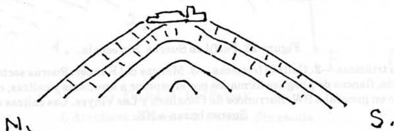
Figura 26. Anticlinal en el sendero de Tales a Sueras. Bóveda de la charnela de calizas del Muschelkalk. Sin escala.
