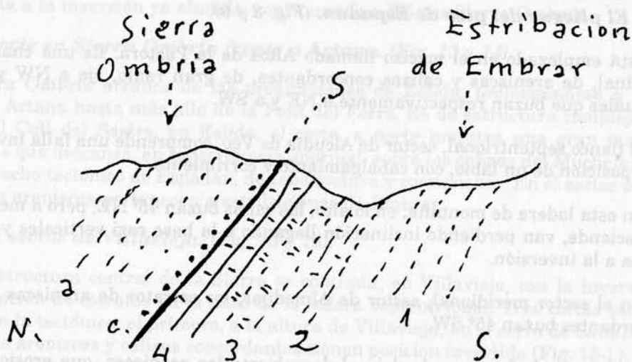
Figura 7. Cabalgadura brechoide, milonito, en las alturas del Coll del Sastre. Eslida. 1. Areniscas del nivel superior del Buntsandstein, de rodenos rojos. — 2. Areniscas vinosas. — 3. Capas de paso a las calizas. — 4. Calizas del Muchelkalk grises y ferruginosas. — 5. Superficie de cabalgamiento y milonito. — c. Conglomerado de base del Buntsantstein, en posición anómala de cabalgamiento. — a. Areniscas, rodenos, de la base del Triásico. Sin escala.
