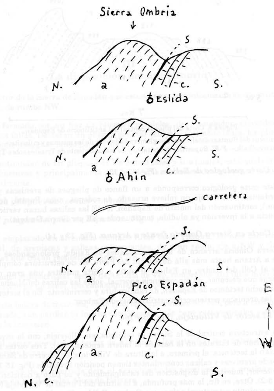
Figura 9. Cabalgamiento, sector Pico de Espadán, prolongación E, hasta Sierra Ombría.
