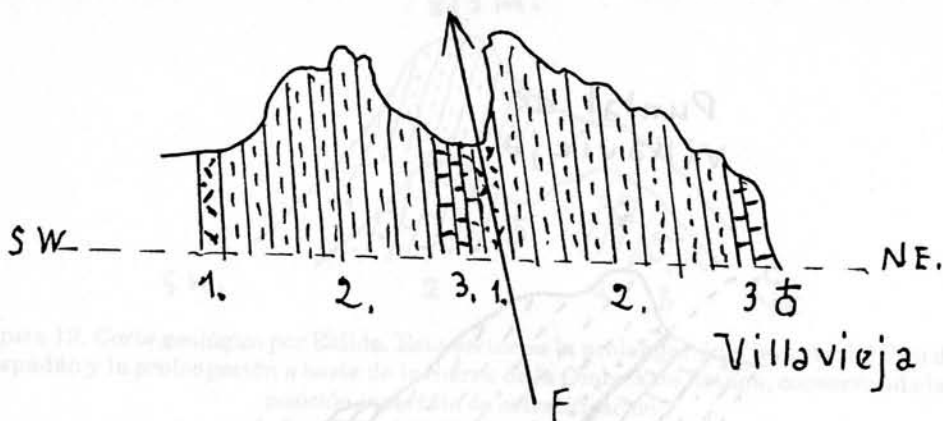
Figura 16. Corte en la terminación de Espadán en Villavieja.
