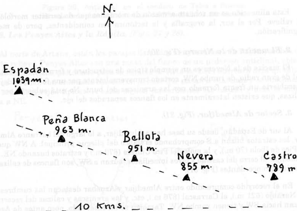
Figura 29. Relieve del sector meridional del anticlinorio.
