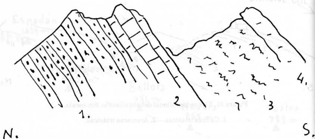
Figura 33. Desde Almedijar a Azuébar antes de llegar al pueblo. Sin escala 1. Areniscas del Triásico.—2. Calizas del Triásico.—3. Margas del Keuper.—4. Carniolas. En este perfil aparece la serie completa del Triásico.
