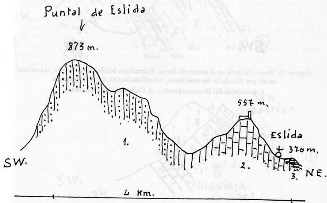
Figura 11. Corte por el Punta de Eslida.
