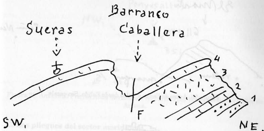
Figura 23. Perfil de Sueras. Sin escala.
