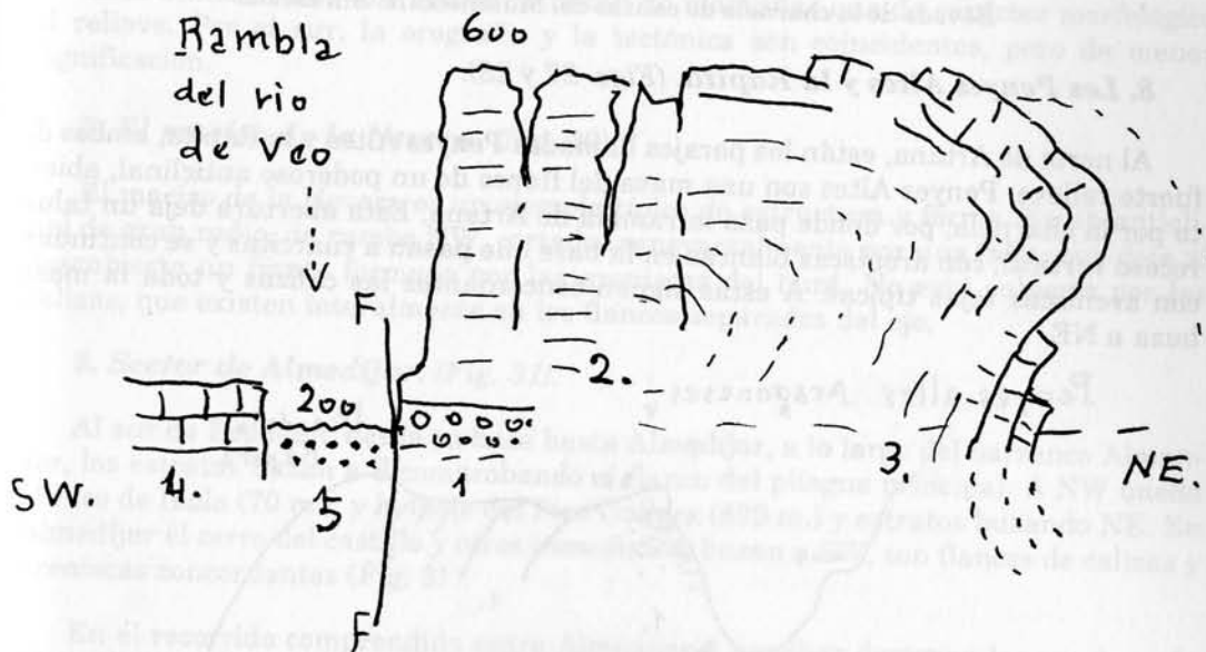
Figura 24. Falla de Benitandús, parte de la charnela de un pliegue anticlinal. Sin escala.
