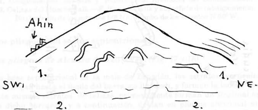
Figura 19. Anticlinal en los corrales de Ahín.
