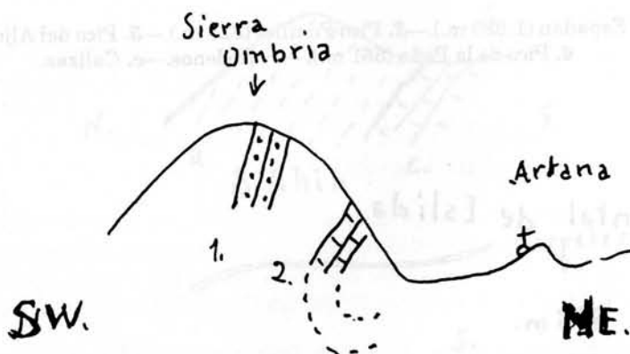
Figura 13. Sierra Ombría en el sector de Jorva. Estructura tectónica invertida, las calizas están por debajo de las areniscas, las calizas buzan 45^{\circ} S. Sin escala.
