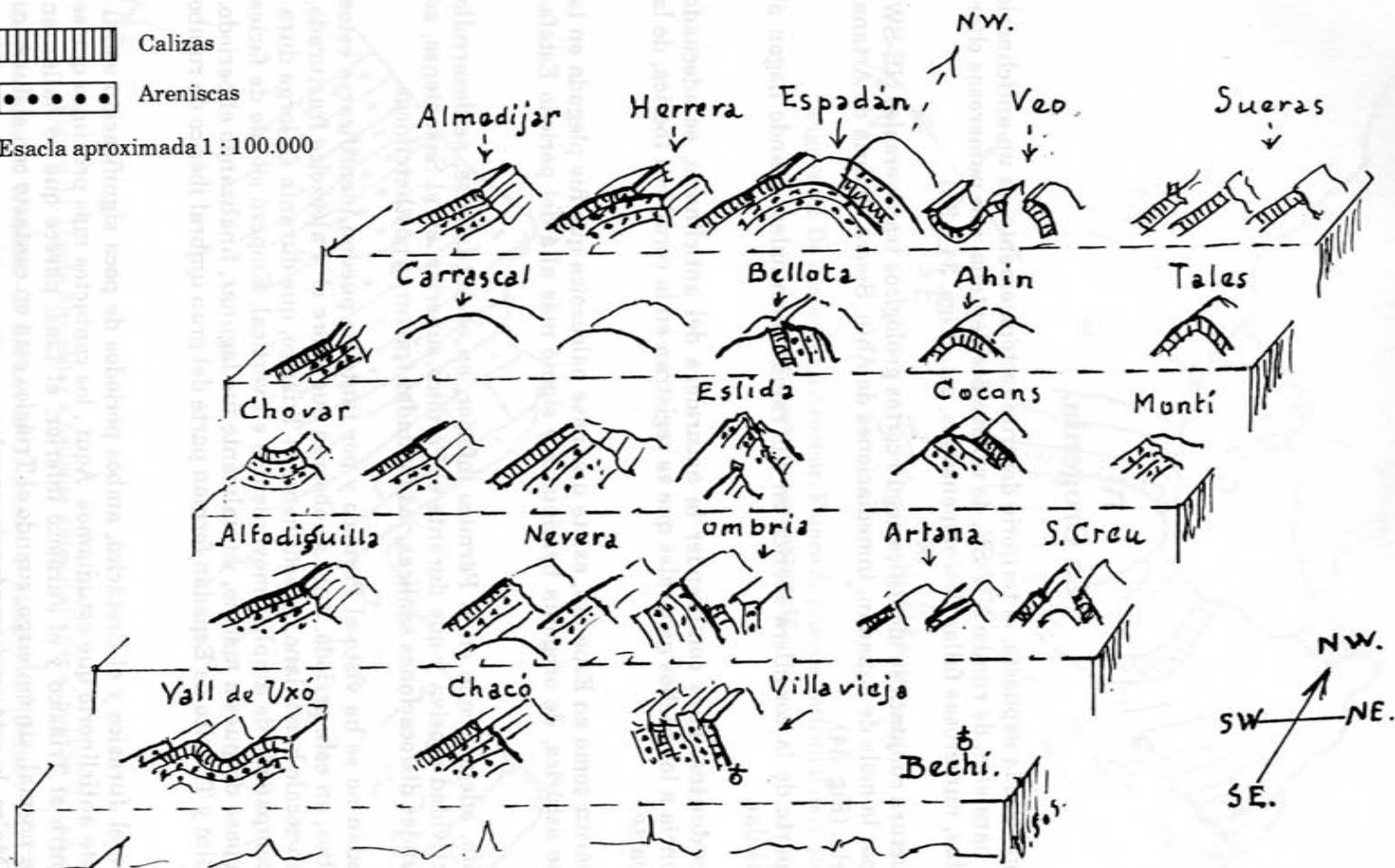
Figura 34. Bosquejo del anticlinorio de la Sierra de Espadán.
