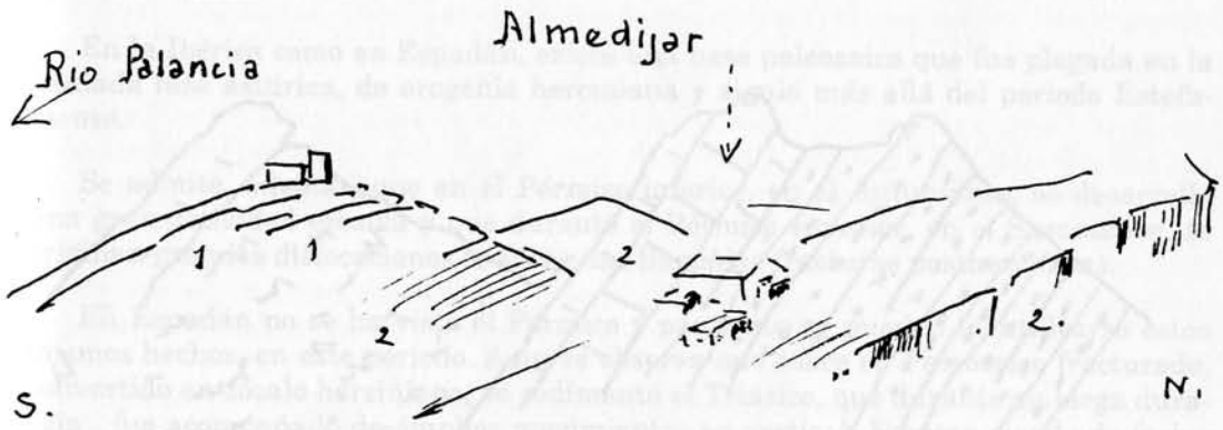
Figura 31. Flanco meridional del anticlinorio. Sin escala.
