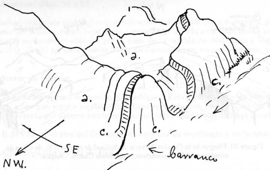
Figura 32. De Almedijar a Azuébar. Flanco de pliegue anticlinal partido, con fuerte buzamiento a SE.
