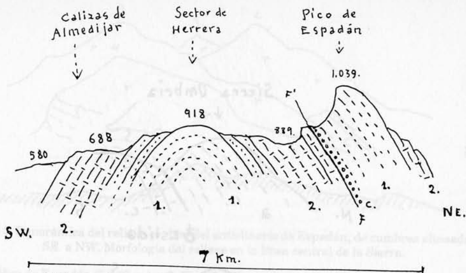
Figura 8. Corte del pliegue central del anticlinorio de Espadán.
