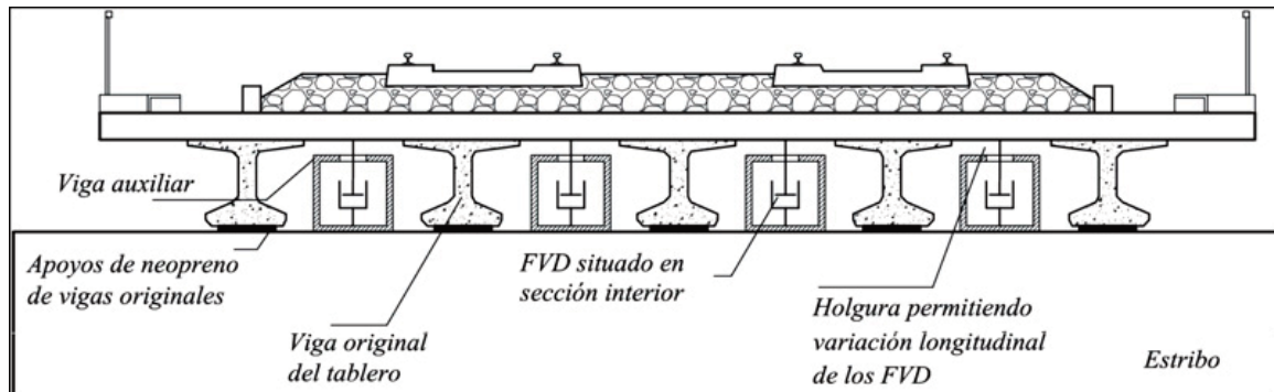
Figura 1. Sistema de reacondicionamiento propuesto instalado en tablero de vigas
