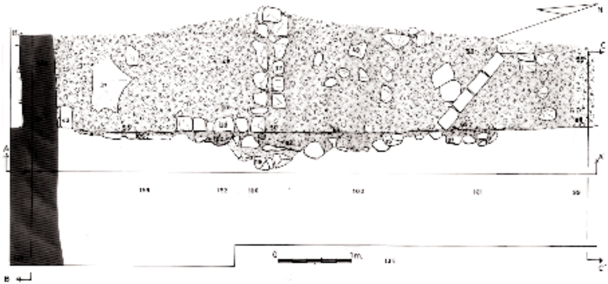
Fig. 3. Planimetría de la muralla.
