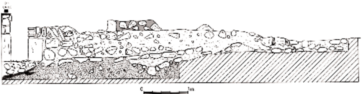
Fig. 4. Alzado de la muralla.
