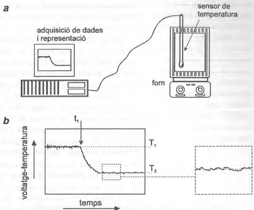
Fig. 2.1 Enregistrament de la temperatura d'un forn per mitjà d'un sensor de temperatura i un sistema d'adquisició de dades i representació. El sensor converteix la temperatura en un senyal de voltatge amb retard temporal negligible. El forn es troba inicialment a temperatura T_1 , i en l'instant t_1 s'ha abaixat a T_2 per mitjà del regulador: (a) esquema del muntatge; (b) ampliacions de les dades de temperatura enregistrades, on es veu la corba després de t_1 a causa del temps d'estabilització del forn.
