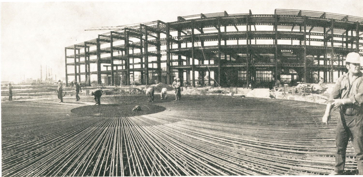
La Central Térmica en construcción
