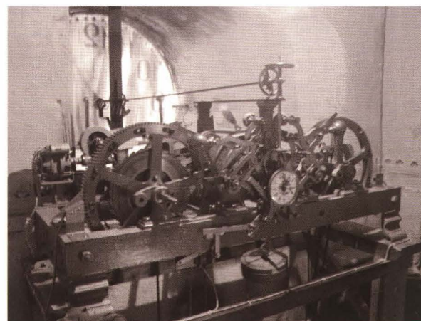
"Maquinària de l'actual rellotge del campanar encara amb algunes peces originals"
