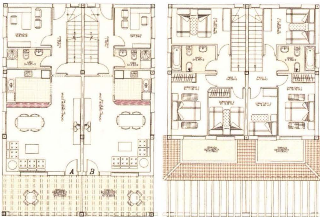
PLANTA BAJA
