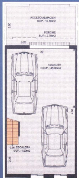
semisótano
