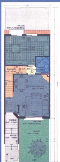
planta baja
