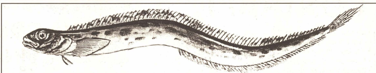
PECECILLO. Ejemplar dibujado de Lumpeno, pez que habita en nuestras costas.
