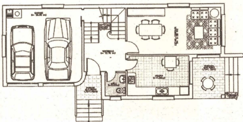
PLANTA BAJA
