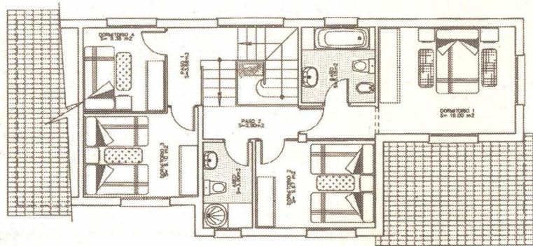
PLANTA PRIMERA
