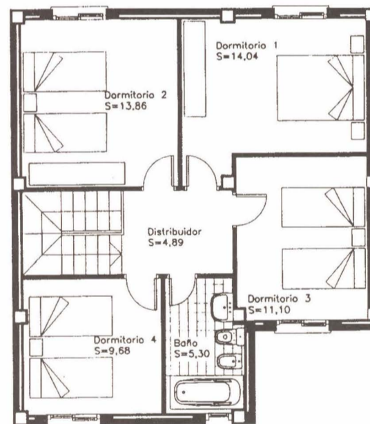
PLANTA PRIMERA Superficie construida por vivienda 73,36 m 2 .
