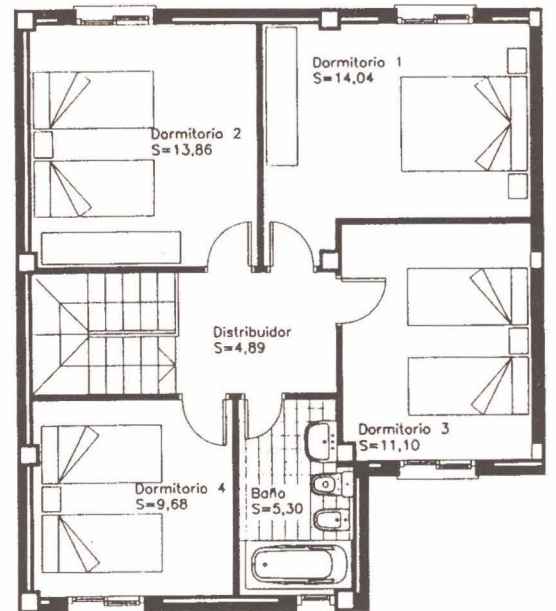
PLANTA PRIMERA Superficie construida por vivienda 73,36 m2.
