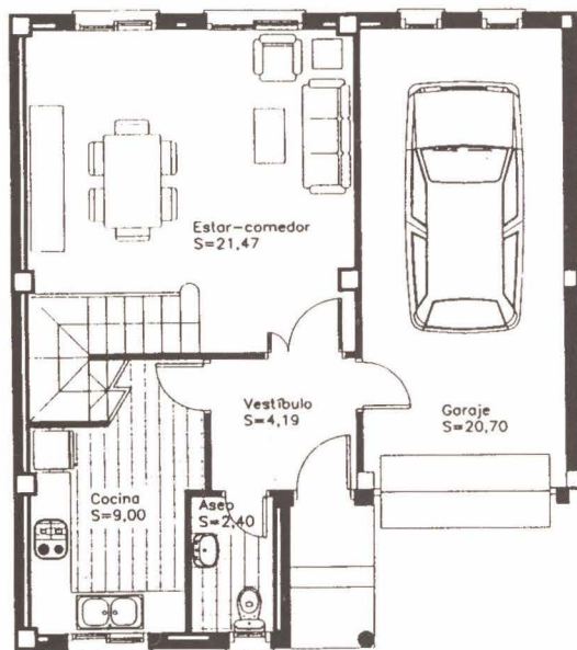
PLANTA BAJA Superficie construida por vivienda 70,21 m2.
