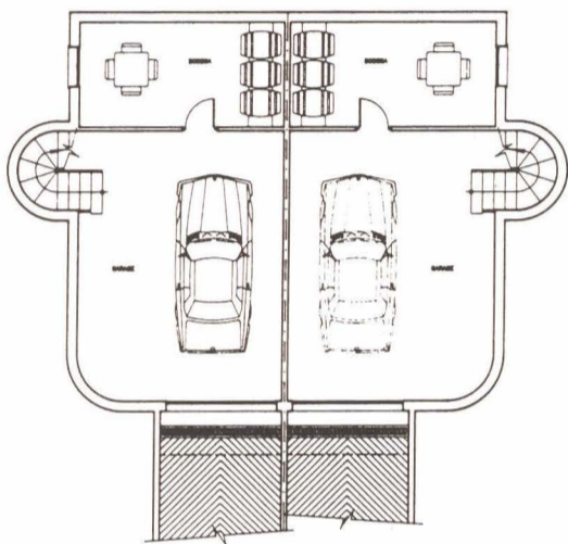
PLANTA SEMISÓTANO
