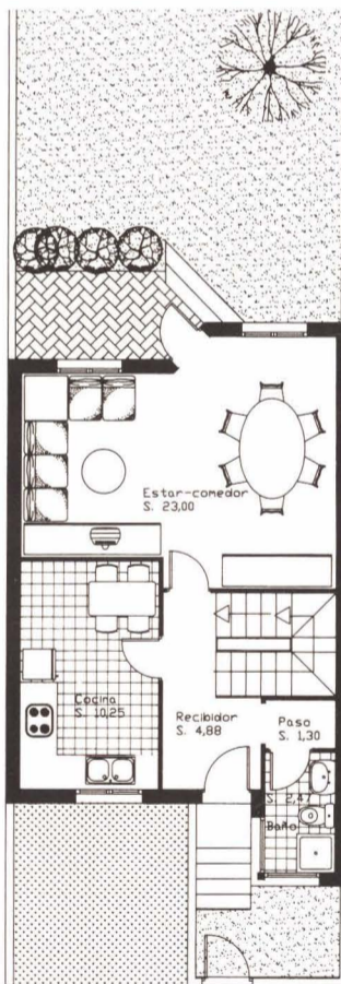
PLANTA BAJA SUP. 56'56
