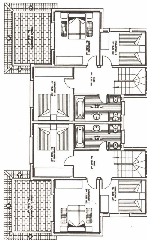
PLANTA PRIMERA
