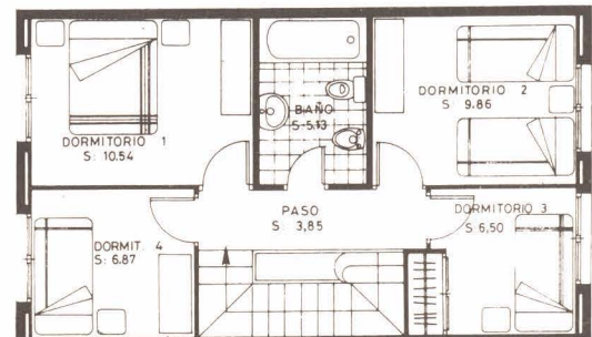
PL. PRIMERA
