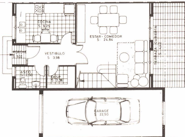
PL. BAJA
