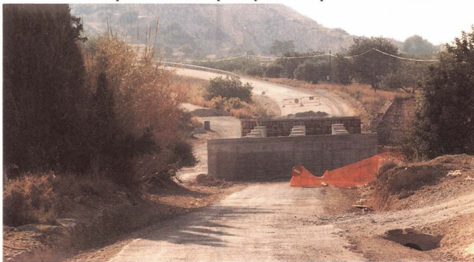
Avançades les obres del pont de la carretera entre Vinaròs i Càlig. Foto: Reula
