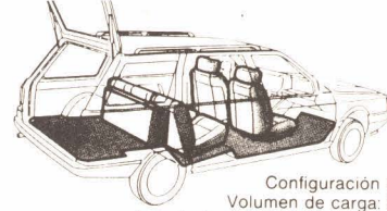
Configuración 2 plazas Volumen de carga: 1.694 dm 3 Longitud máxima de la carga: 1.705 m.
