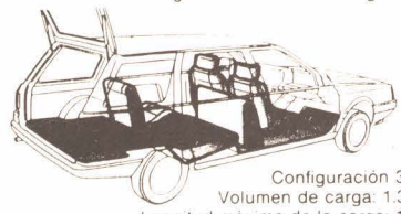
Configuración 2 plazas Volumen de carga: 1.710 dm 3 Longitud máxima de la carga: 1.745 m.
