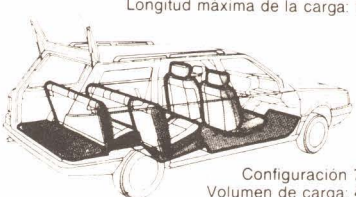
Configuración 5 plazas Volumen de carga: 922 dm 3 Longitud máxima de la carga: 1.010 m.
