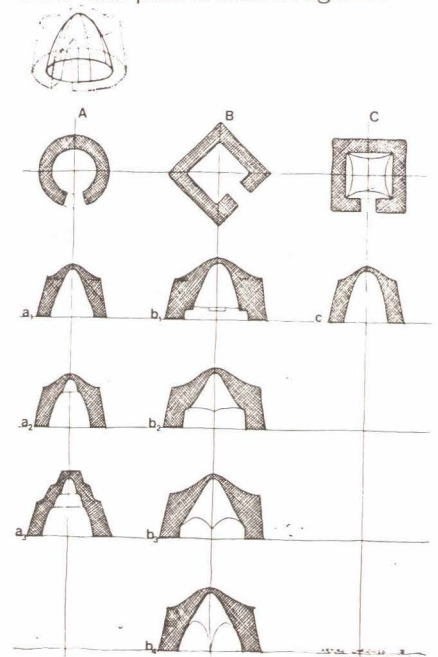
Tipus de barraques de pedra en sec segons la forma de la volta. Segons Arturo Zaragoza
