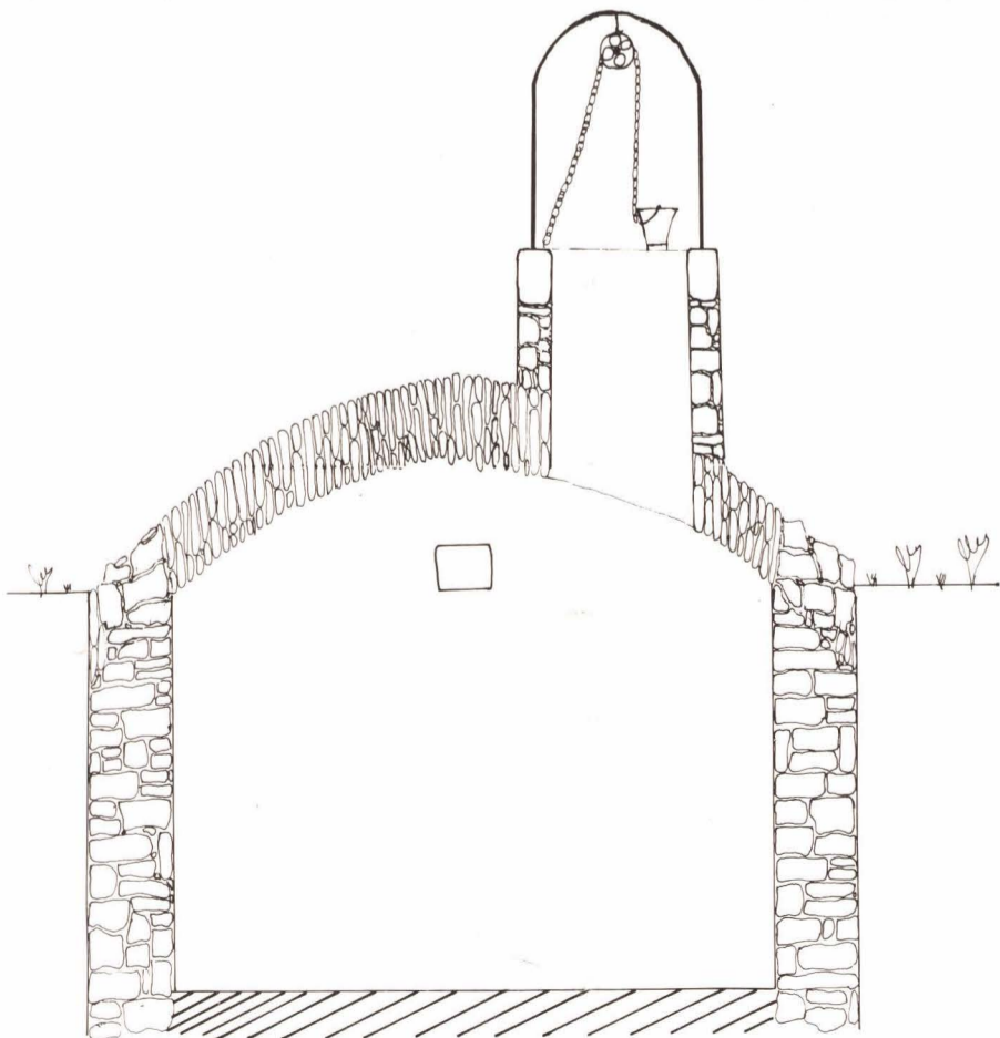
Sección de un aljub
