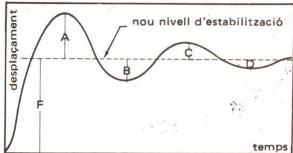
Resposta d'un sistema subcrític a una pertorbació brusca (factor d'amortiment = F/A , A/B , B/C , etc)
