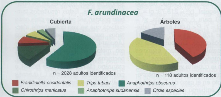
Figura 3. Composición específica de trips en cada uno de los sistemas de gestión del suelo considerados en este estudio.
