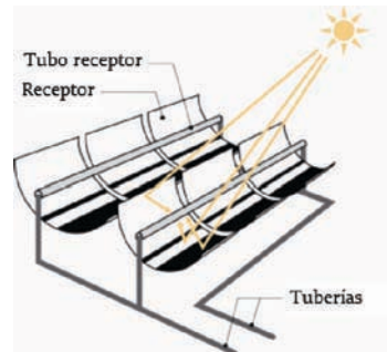
Figura 1.2: Central de cilindro parabólico.
