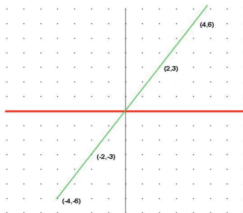
Figura10. Representación de algunos pares de la clase de equivalencia de (2,3)
