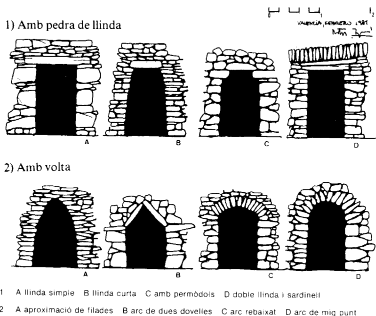
Figura 3.1.D. Tipus d'embocadura en barraques.
