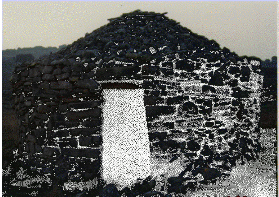
FOTO 2: Planta circular. Murs verticals i arranc de la cúpula molt alts. Porta a triple llinda amb gravats. Carreus de la porta molt regulars. Pla de Vistabella.
