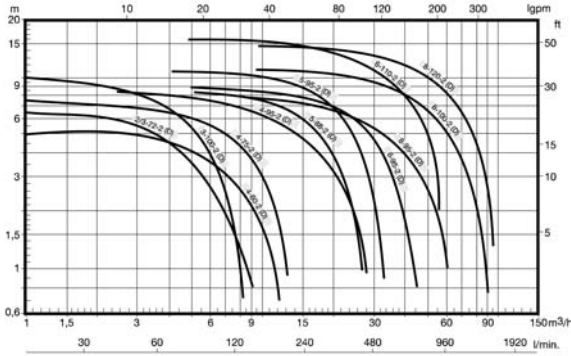
CAMPO DE TRABAJO a 2.800 r.p.m.
