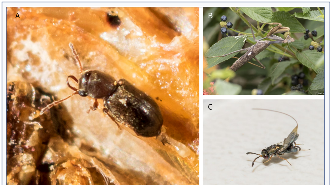
FIGURA 1. A: Imago macho de Ozognathus cornutus (LeConte, 1859) (Ptinidae); B: Imago de Sphodromantis viridis (Forskål, 1775) (Mantidae); C: Imago hembra de Podagrion splendens Spinola, 1811 (Torymidae). Autor de las fotografías: Jorge Herrero-Hernán.
