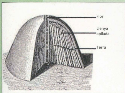
Esquema d'una carbonera.
