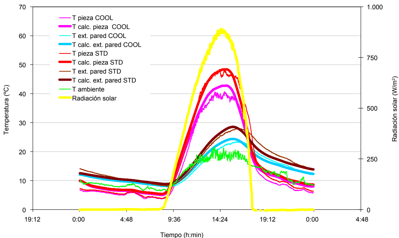
Figura 9. Validación de las temperaturas simuladas frente a los datos experimentales monitorizados para un día de invierno (8 de enero).
