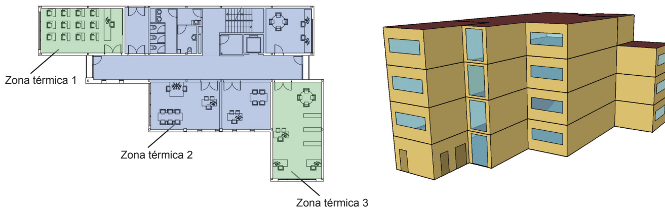
Figura 8. Esquema planta edificio CIES (izquierda) y edificio CIES modelizado (derecha).
