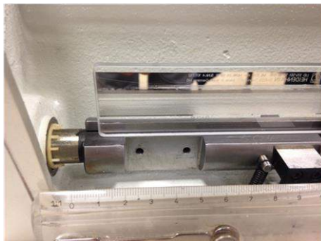
Figura 2: Al desmontar la máquina, se observó que el problema se encontraba en la deslizadera principal. La regla óptica (la parte más sensible) estaba dañada. Se pueden ver los arañazos en la imagen.
