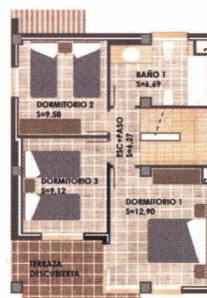
PLANTA PRIMERA Superficie construida 54,04 m
