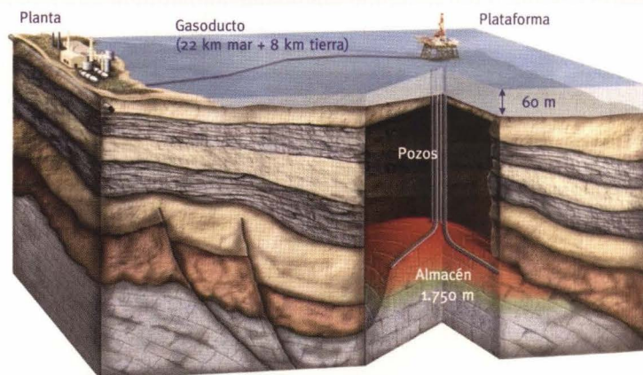
Esquema general de les instal·lacions
