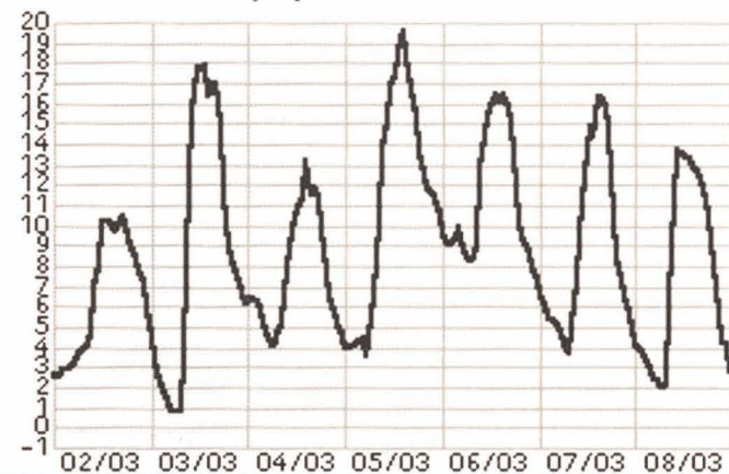
RAFEGA MÀXIMA DE VIENTO (kmh) - to mar 08 2005
