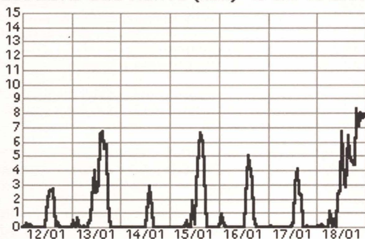
VELOCIDAD DEL VIENTO (kmh) - to ene 18 2005
