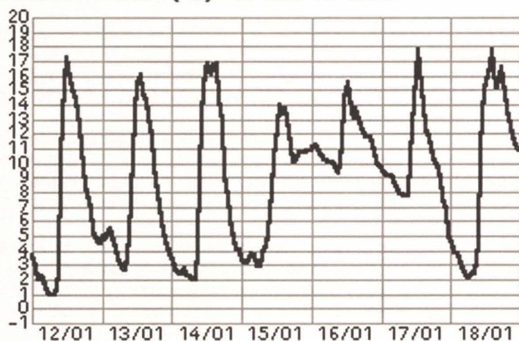
TEMPERATURA (°C) - to ene 18 2005
