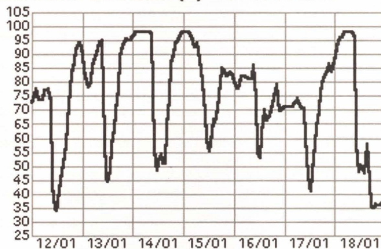
HUMEDAD RELATIVA (%) - to ene 18 2005
