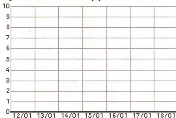
Daily PRECIPITACIONES (L) - to ene 18 2005
