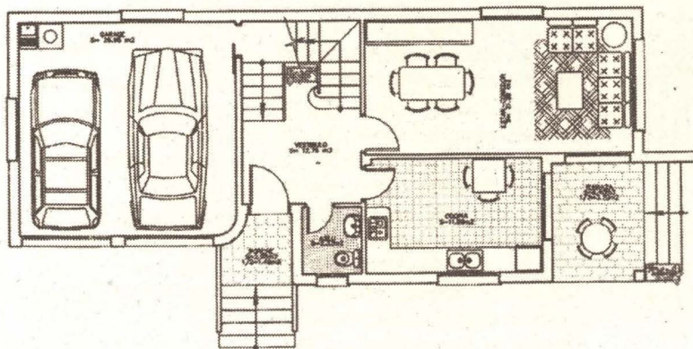
PLANTA BAJA
