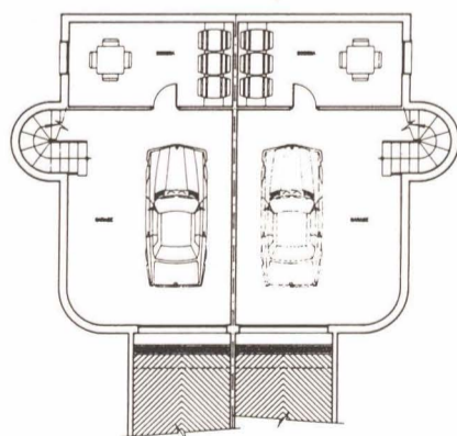
PLANTA SEMISÓTANO
