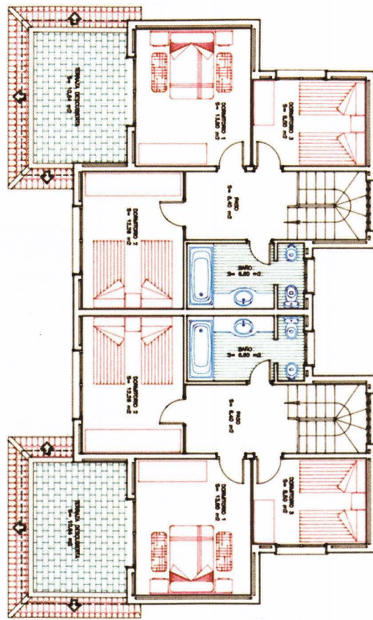
PLANTA PRIMERA
