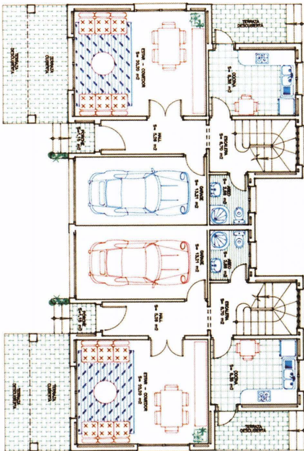
PLANTA BAJA
