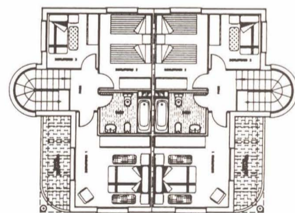
PLANTA PRIMERA
