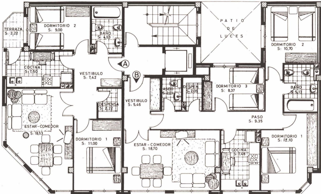
PLANTA DISTRIBUCION.
