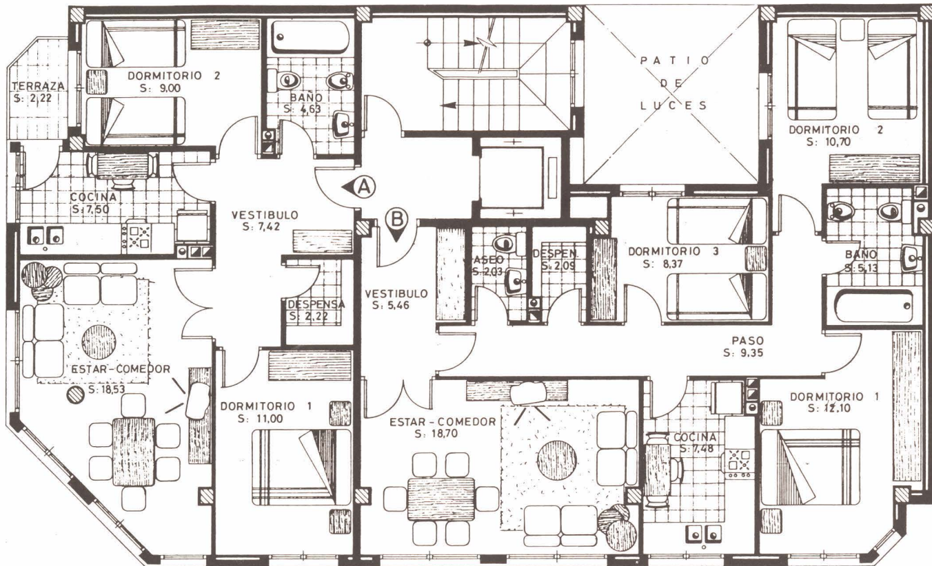
PLANTA DISTRIBUCION.
