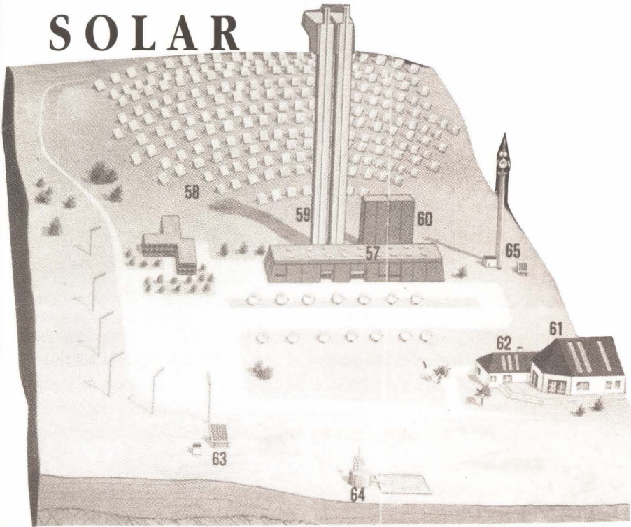
En las centrales electrosolares (57), la radiación, recogida en espejos colectores orientables –heliostatos (58)–, se refleja y concentra en calderas colocadas en lo alto de las torres (59). Allí calienta un fluido que, mediante un intercambiador, cede sus calorías al agua. El vapor hace girar una turbina que acciona un alternador (60). Los paneles de los tejados (61) aseguran la calefacción. Las pilas fotovoltaicas transforman la energía solar en electricidad de usos privados (62) o públicos (63), alimentan bombas de agua (64) y sistemas de telecomunicación (65).
