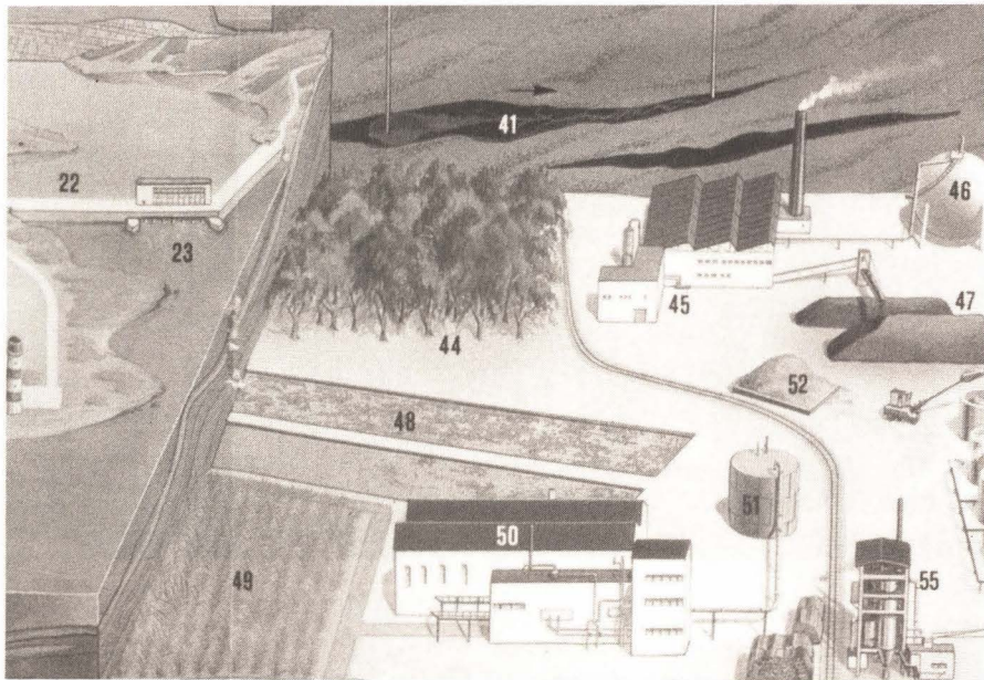
Hay numerosas técnicas de conversión. Se pueden explotar árboles de crecimiento rápido, con el eucalipto (44); la pirolisis-descomposición por el calor y al abrigo del aire (45) proporciona carbón de madera (47) y gases pobres (46). Los jacintos de agua (48) se transforman en metano.
