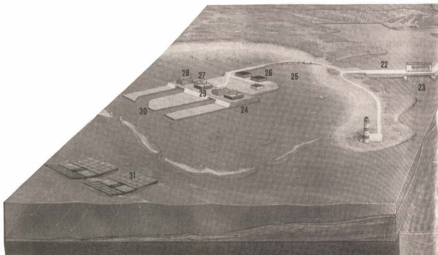
Un dique (22) retiene el agua de la marea alta y la devuelve al mar a través de un grupo turboalternador (23). La energía térmica de los mares cálidos procede de la diferencia de temperatura entre la superficie y las profundidades. Esta central (24) podría estar en Tabiti: es de ciclo cerrado y utiliza un fluido intermediario, el amoníaco. El agua caliente (25), bombeada (26), le cede su calor a través de un intercambiador (29); el vapor se detiene en una turbina (28) y pasa al condensador (27) alimentado por agua de mar fría. El agua caliente es rechazada (30). Las balsas de Cockerell (31) aprovechan la energía de las olas, recogiendo al nivel de las articulaciones por medio de bombas hidráulicas.
