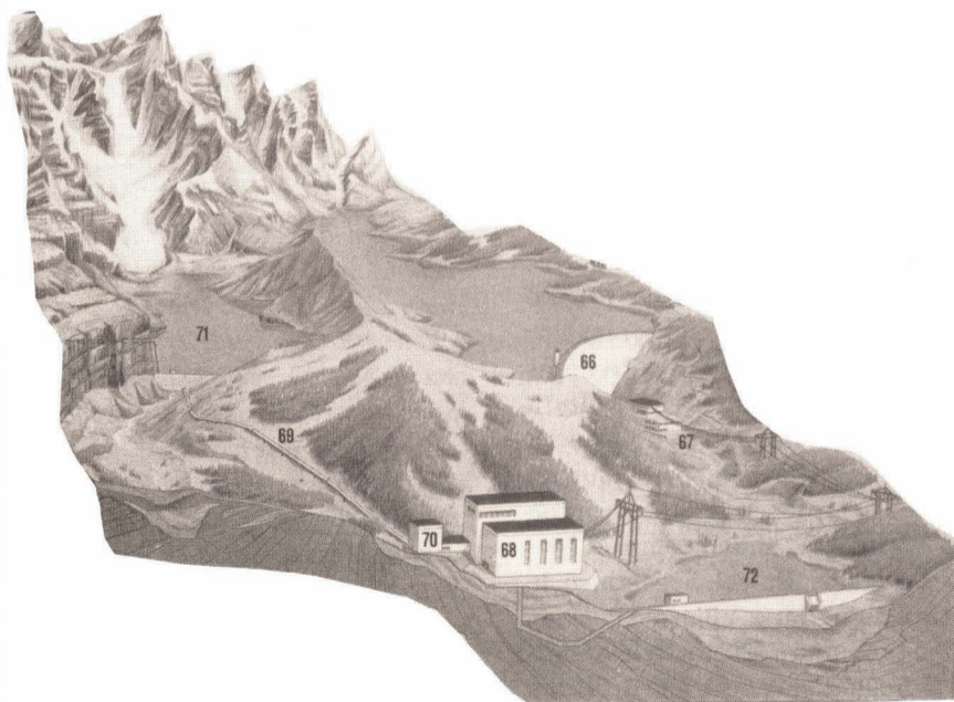
Las presas (66) retienen masas de agua a nivel elevado. Cuando llega al nivel inferior, el agua acciona la turbina de la central (67). Las centrales de bombeo (68), equipadas con compuertas dobles (70), permiten el reciclamiento continuo. El agua es transportada hasta allí mediante tuberías (69). En boras de poco consumo, el agua del embalse inferior (72) se bombea hacia el embalse superior (71). En las boras punta, recorre el camino inverso, generando electricidad (73).
