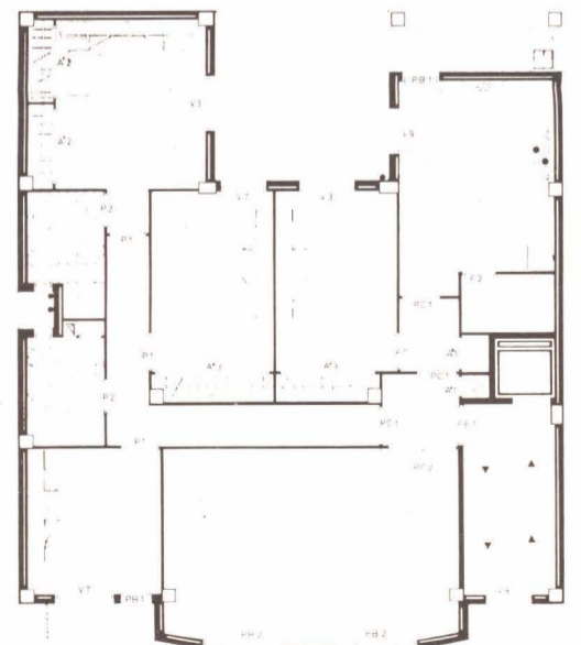
PLANTA PISOS
