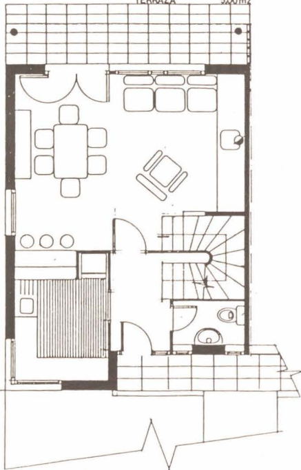
PLANTA BAJA
