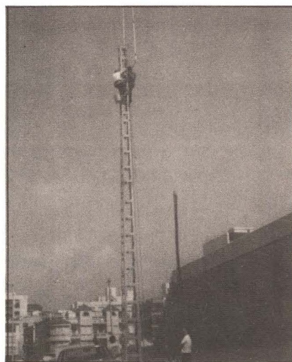
Terminada la instalación definitiva de las dos antenas sobre una altura aproximada de doce metros. Fotos tomadas en el puerto de Vinaròs el día 24-6-84.
