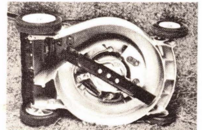
CARTER AERODINAMICO
