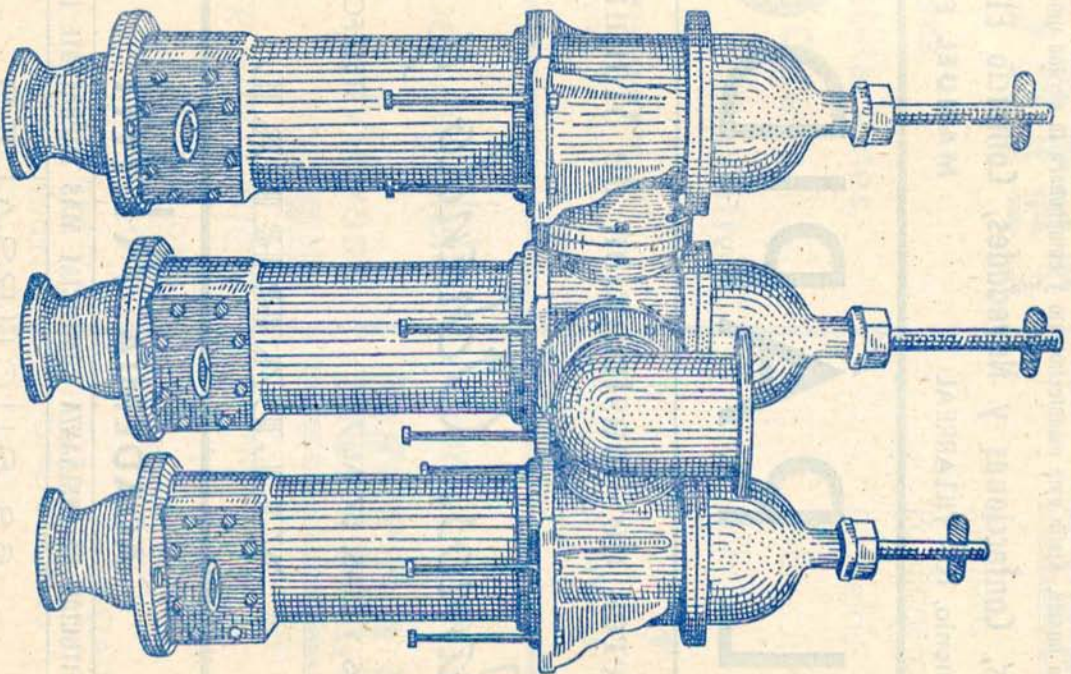
CUERPO TRIPLE DE BOMBAS DE PISTÓN
