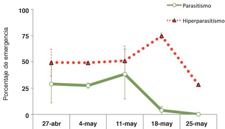
Figura 7. Dinámica estacional del parasitoides primario B. angelicae y sus hiperparasitoides emergidos (porcentaje medio de emergencia ± EE) de las momias de A. spiraecola recolectadas en cuatro parcelas de clementinos en 2012 y 2013 (modificado a partir de Gómez-Marco et al. , 2015).
