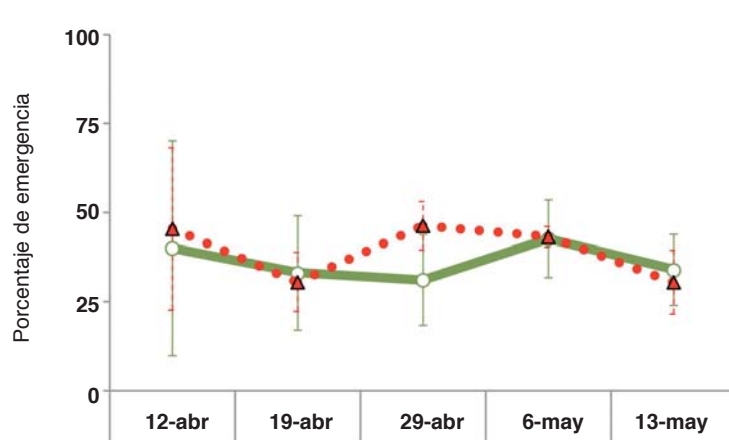
Figura 7. Dinámica estacional del parasitoides primario B. angelicae y sus hiperparasitoides emergidos (porcentaje medio de emergencia ± EE) de las momias de A. spiraecola recolectadas en cuatro parcelas de clementinos en 2012 y 2013 (modificado a partir de Gómez-Marco et al. , 2015).
