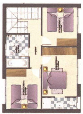
VIVIENDA TIPO 2 SUPERFICIE UTIL=85,00m 2 SUP.CONSTRUIDA=100,00m 2
