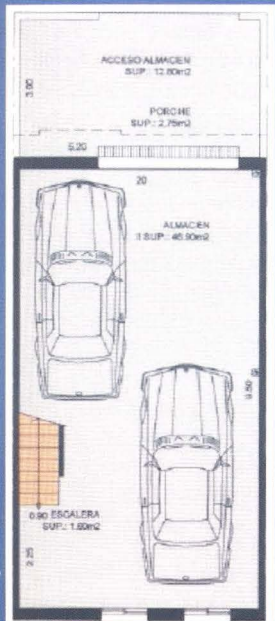
semisótano
